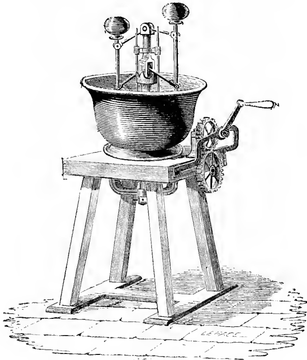
PULVERISER.
